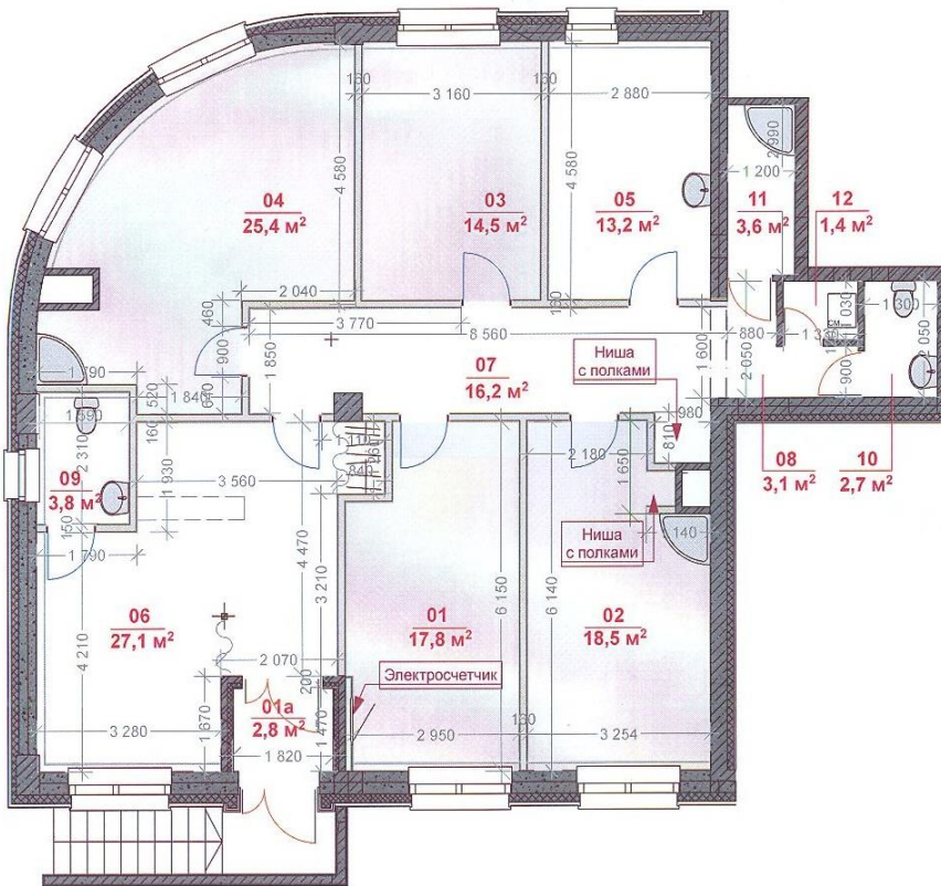
Помещение №VIII (М 1:100)
