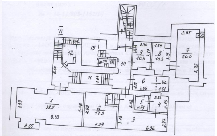
план подвала
