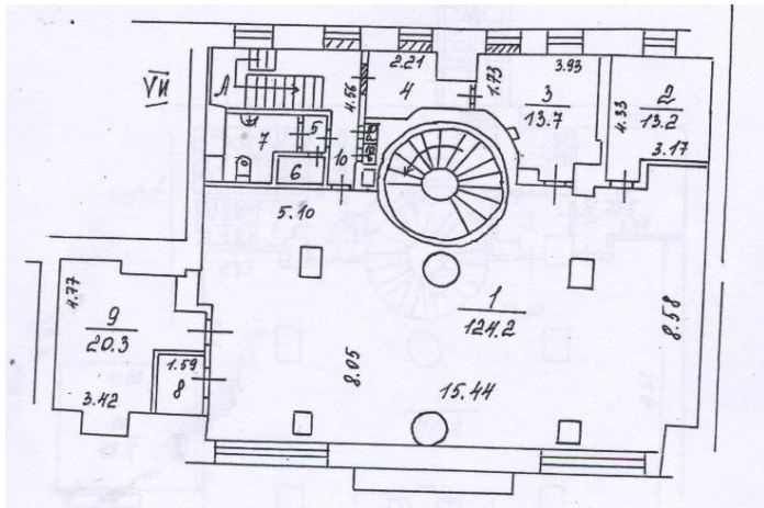
План 2-ого этажа
