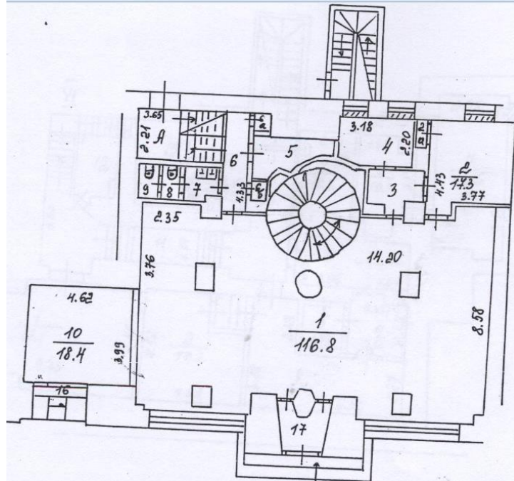
План 2-ого этажа
